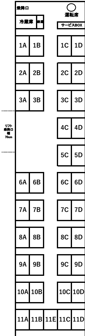
乗降のみ【正シート41席】
